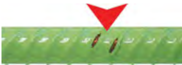
Daño causado por un cabezal para vibrador de acero estándar
